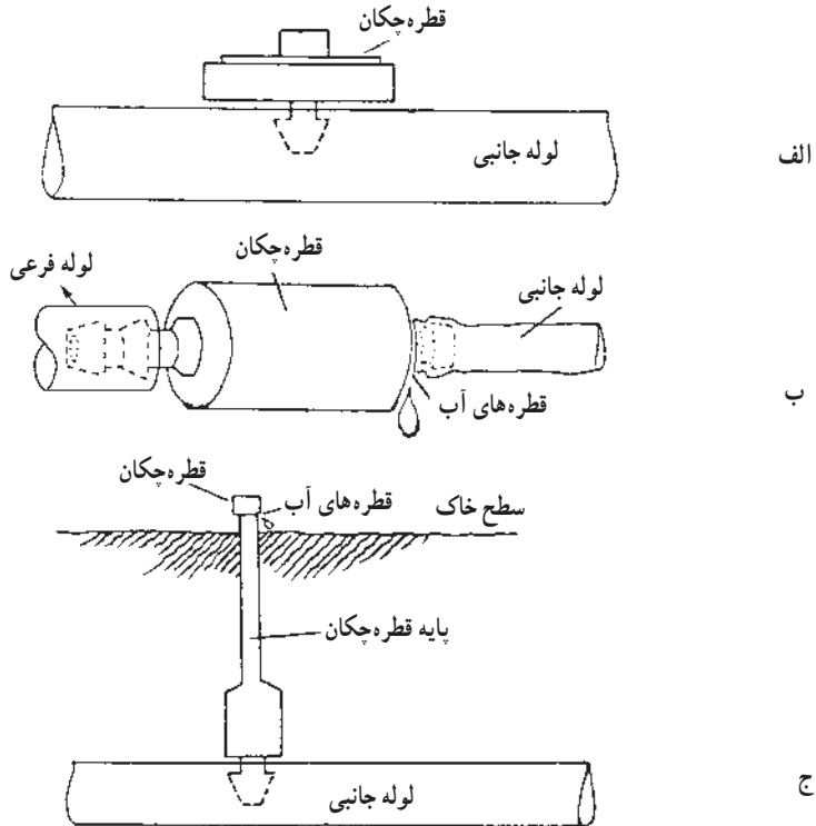
شکل ۶-۱۳ — روش‌های اتصال قطره‌چکان‌ها
